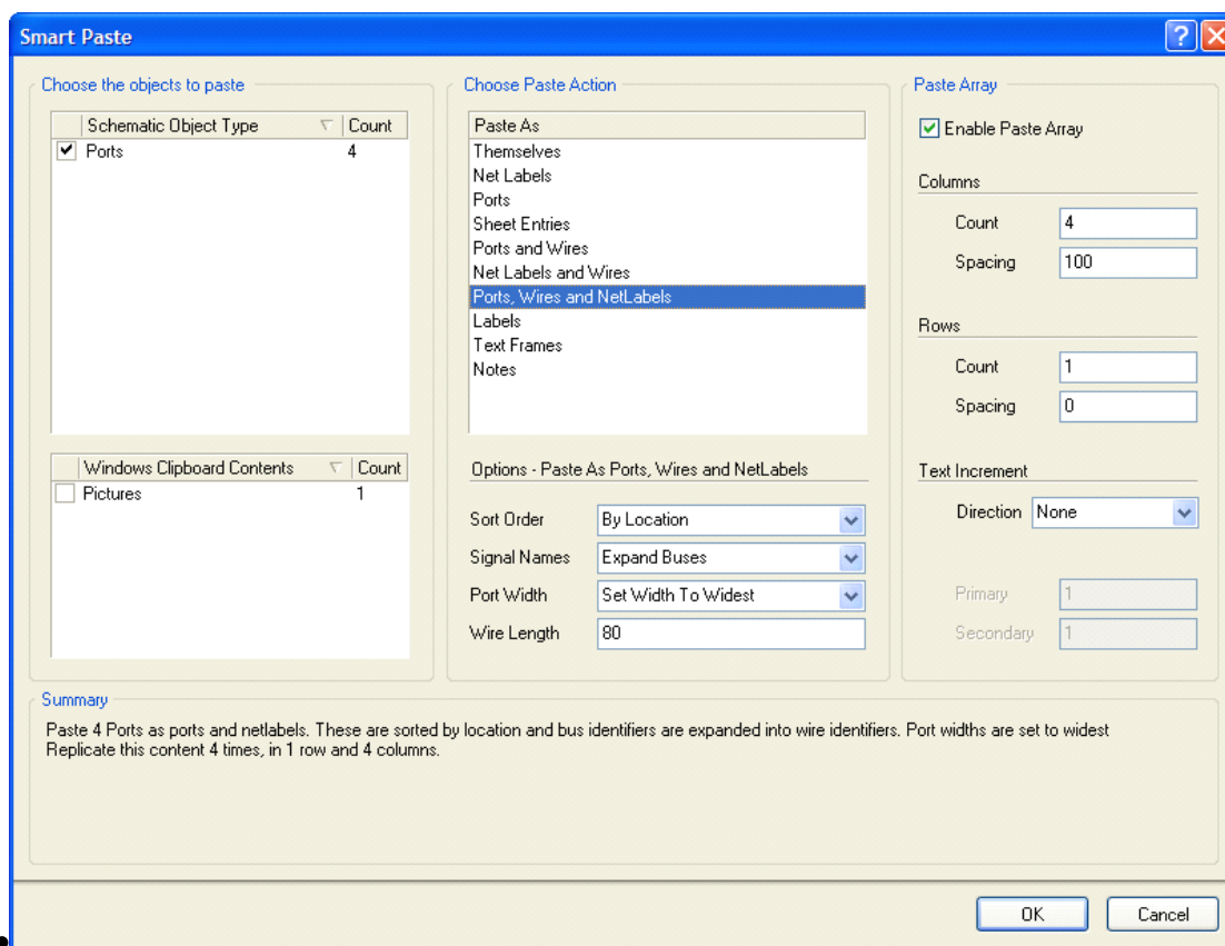
图 53：智能粘贴对话框
